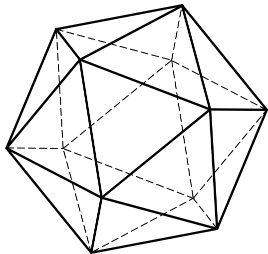
Ikosaeder
