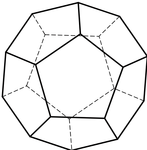
Dodekaeder
